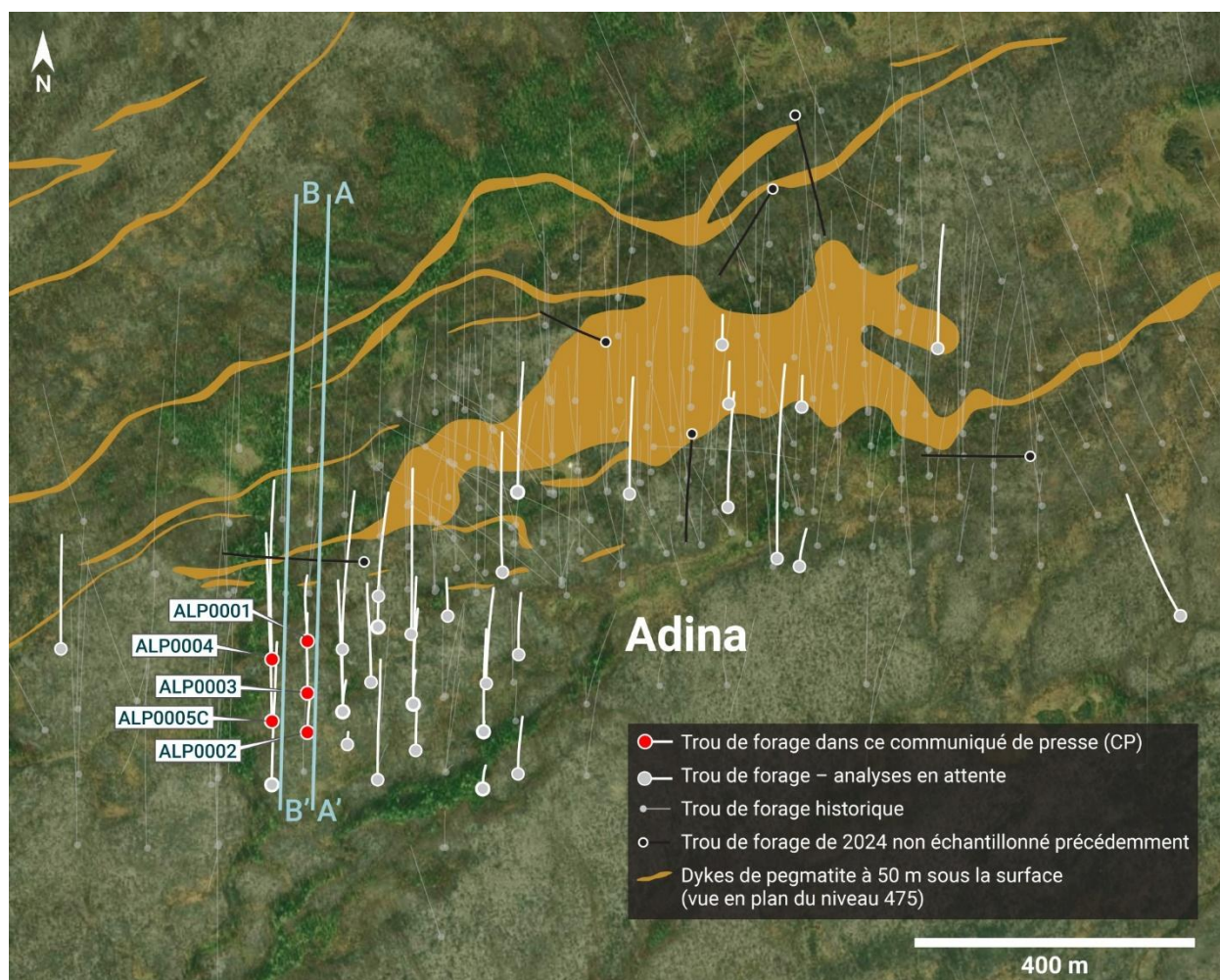
Figure 2 – Plan cartographique montrant les traces de forage historiques et les trous de forage de 2026 de LIFT, ainsi qu'un plan de niveau du complexe de pegmatite Adina-Galinée à 475 m au-dessus du niveau de la mer, soit environ 50 m sous la surface et 25 m sous l'interface roc-till.
