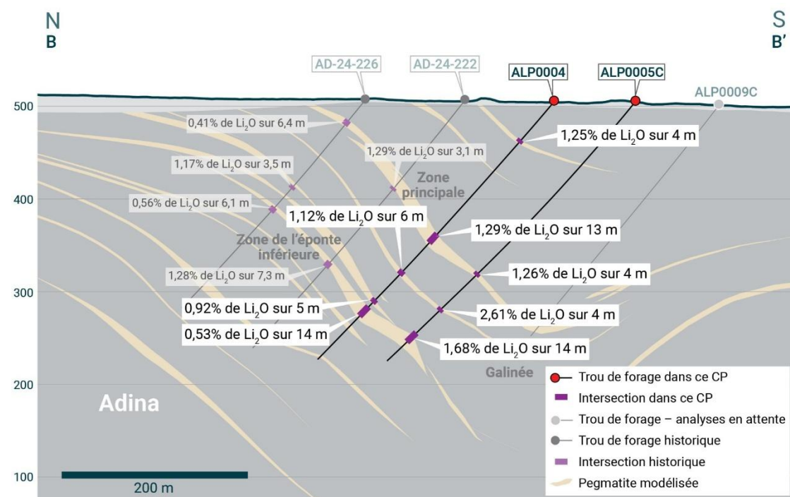
Figure 4 – Coupe vertical nord-sud à travers le complexe de pegmatite Adina-Galinée montrant les résultats de forage de LIFT pour 2026 et les résultats de forage historiques précédemment signalés à l'ASX 7 . La coupe B-B' est illustrée à la figure 2.
